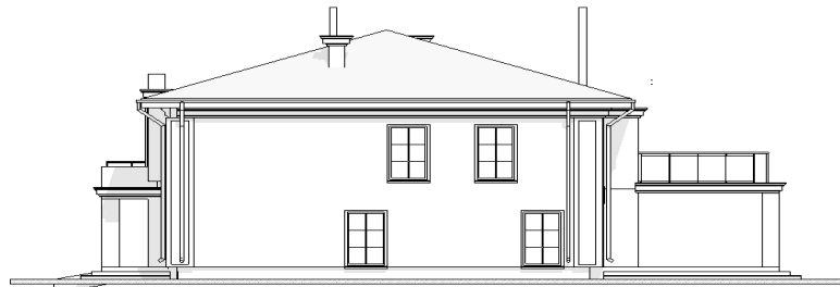
ELEWACJA POŁUDNIOWA
